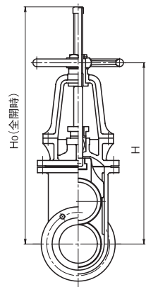
外ねじ式仕切弁
