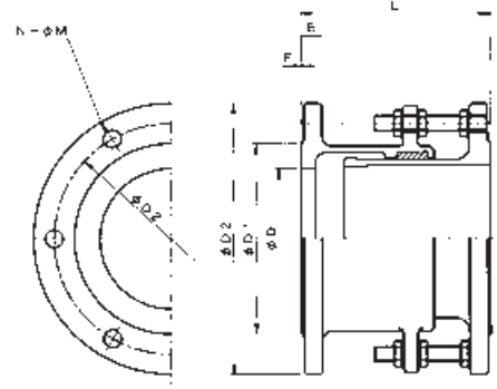
伸縮管
