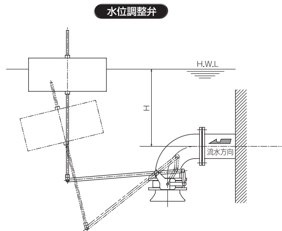
バタフライ式 ステンレス製
