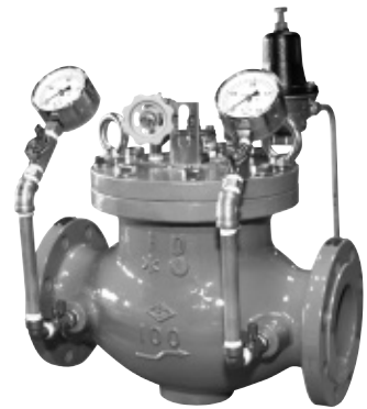
R-2型 減圧弁
