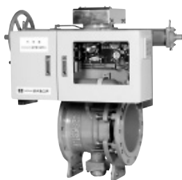
面間伸縮機能付
