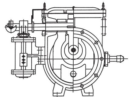
緩閉式(親子弁式)逆止弁
